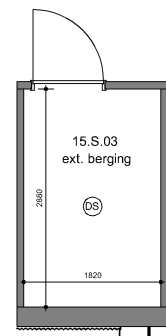
Externe berging, schaal 1:100
